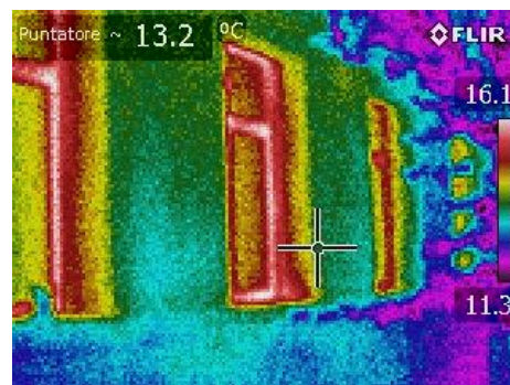
Figura 4 – Rilievo termografico dei serramenti esterni telaio in pvc e vetrocamera – prospetto ovest
